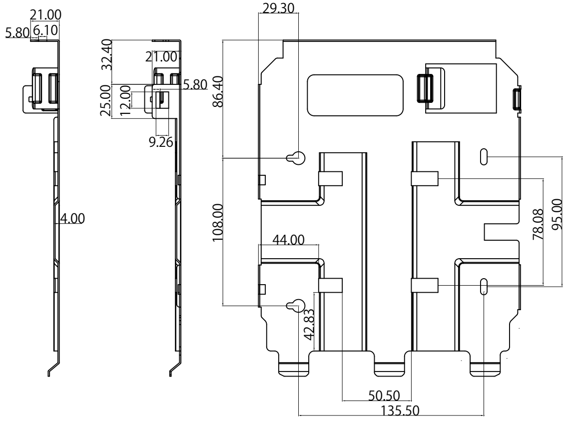
セキュリティカバー用ブラケット
