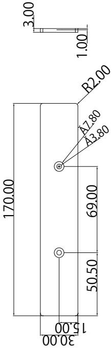
壁掛けプレート
