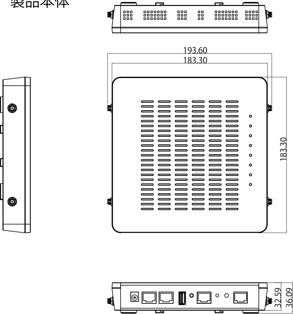
製品本体
