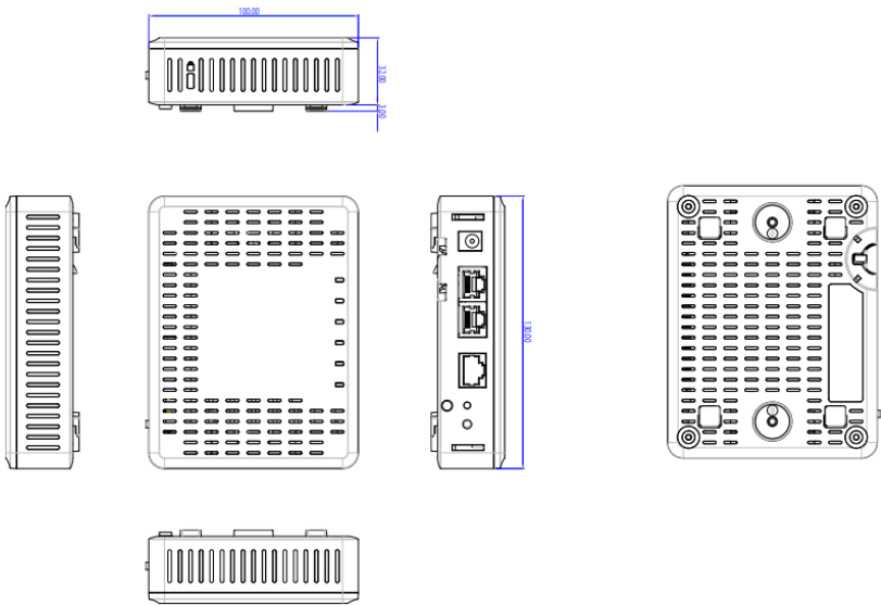
外観図面 型番：WAB-S1775,WAB-S1167
