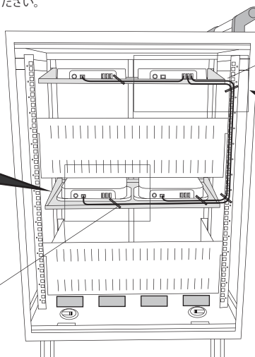
配線用タイ ケーブル固定位置
