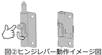
図②ヒンジレバー動作イメージ図
